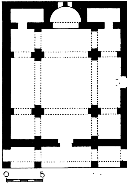
Fig. 1. — SERGIOPOLIS. « L'ÉGLISE EXTRA-MUROS », (d'après E. HERZFELD).
